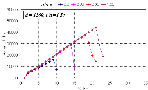
図-3 ペDESTALの寸法比 ( a/d ) の影響
