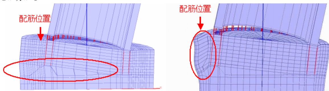
図-1 ペDESTALの特徴的な2種類の破壊モードの例（変形量を200倍に拡大）
