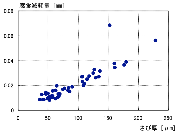
図 3 さび厚と腐食減耗量の関係
