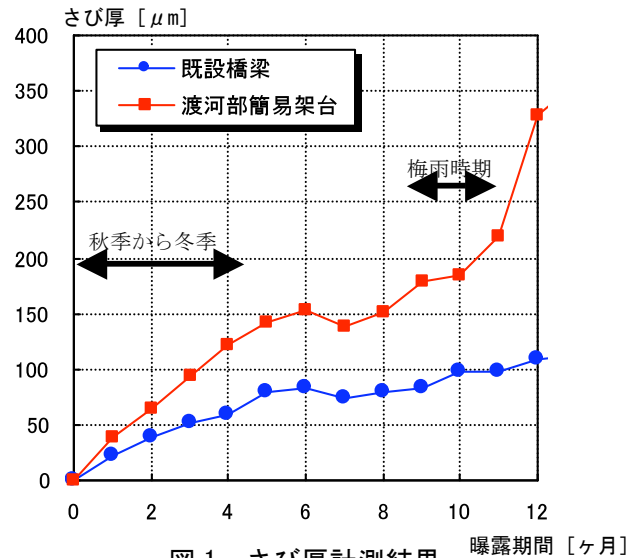
図 1 さび厚計測結果
