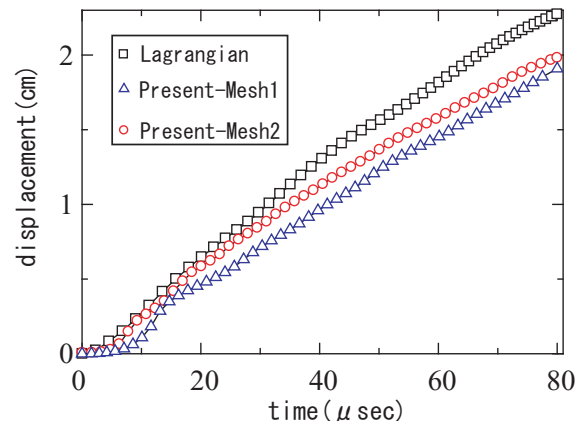
図-8 棒下端部の先端変位の時刻歴
