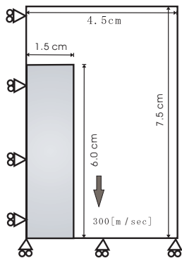
図-3 解析モデル
