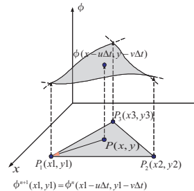
図-1 上流点の評価方法
