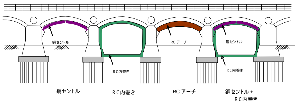
図1 補強工法
