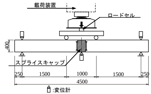
図-4 載荷装置
