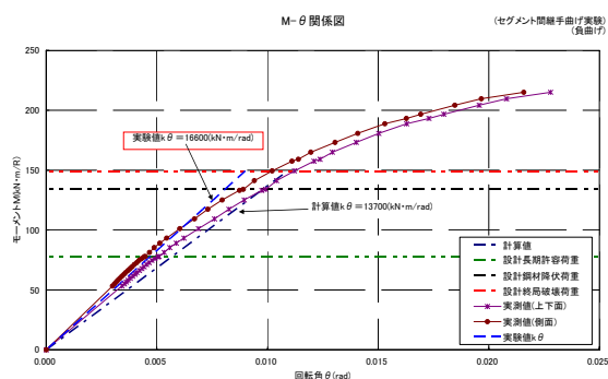
図-6 負曲げ試験結果 ( M-\theta 関係)
