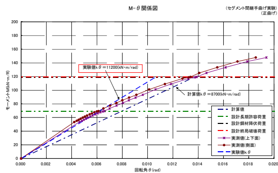
図-4 正曲げ試験結果 ( M-\theta 関係)
