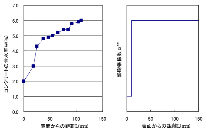
図 2 コンクリートの含水率と熱膨張係数
