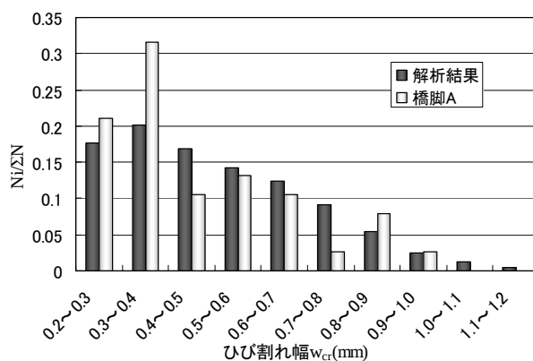
図 7 ひび割れ分布の比較
