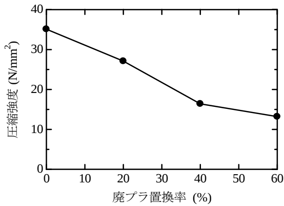
図-2 圧縮強度
