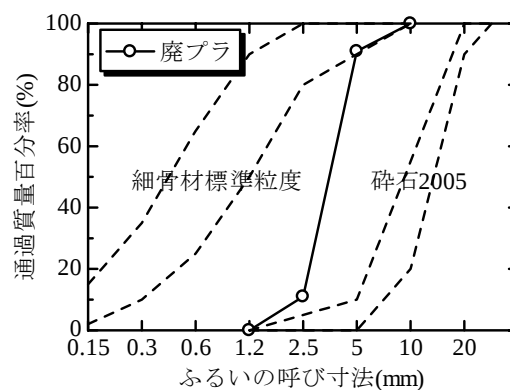
図-1 粒度曲線
