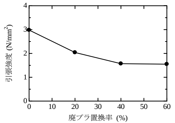
図-3 引張強度
