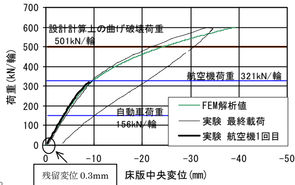
図4 荷重—鉛直変位曲線（一体目）
