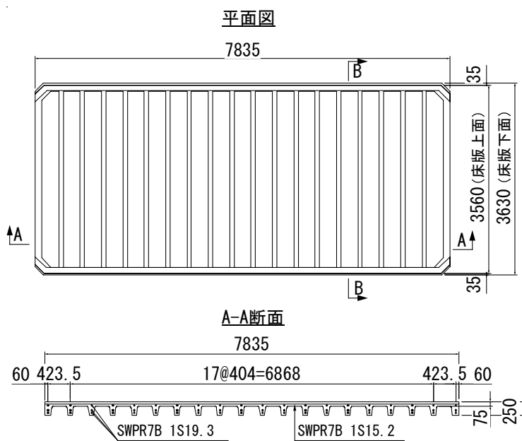
図1 UFC 床版 実物大実験供試体
