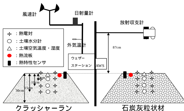
図-1 計測機器配置側面図
