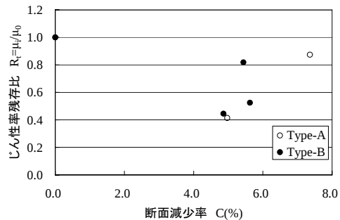
図-8 腐食によるじん性率の低下
