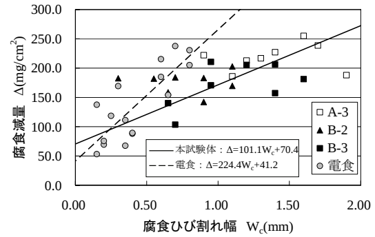
図-6 電食実験との比較
