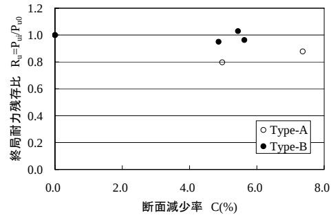
図-7 腐食による終局耐力の低下
