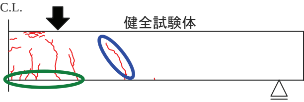
図-3 健全試験体のひび割れスケッチ
