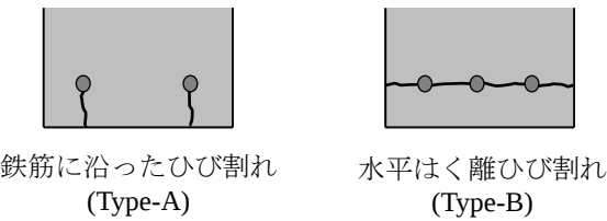
図-2 ひび割れモード
