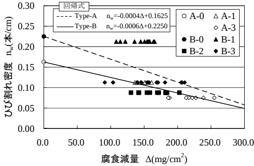
図-5 ひび割れ密度 n_w と腐食減量 \Delta の関係 ひび割れ密度を比較する．ひび割れ密度 n_w は式(1)で定義した．
