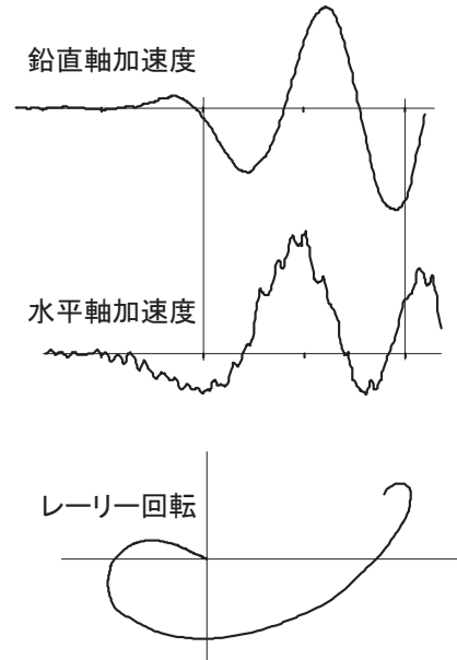
図-3 表面切欠の鉛直と水平の表面弾性波
