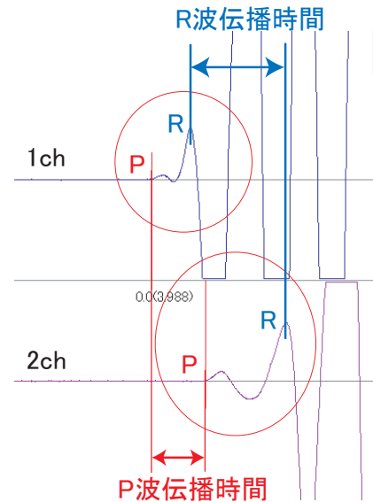
図-1 打点位置と表面弾性波
