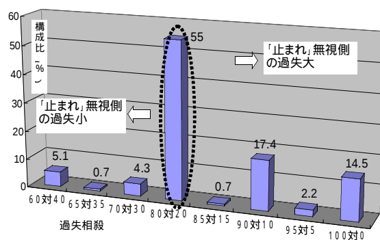
図-2 自動車対自動車の過失相殺
