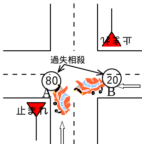
図-1 自動車対自動車の事故
