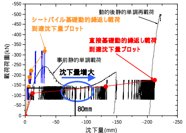
図4 静的載荷と動的繰返し載荷の比較 (荷重—沈下関係)
