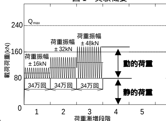
図2 動的繰返し載荷パターン (直接基礎)
