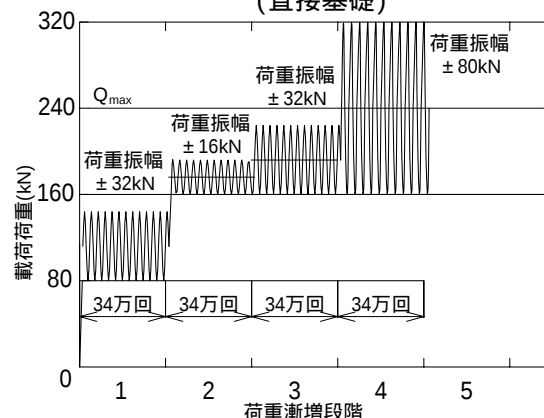
図3 動的繰返し載荷パターン (シートパイル基礎)
