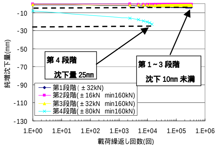
図6 繰返し回数と沈下量の関係 (シートパイル基礎)
