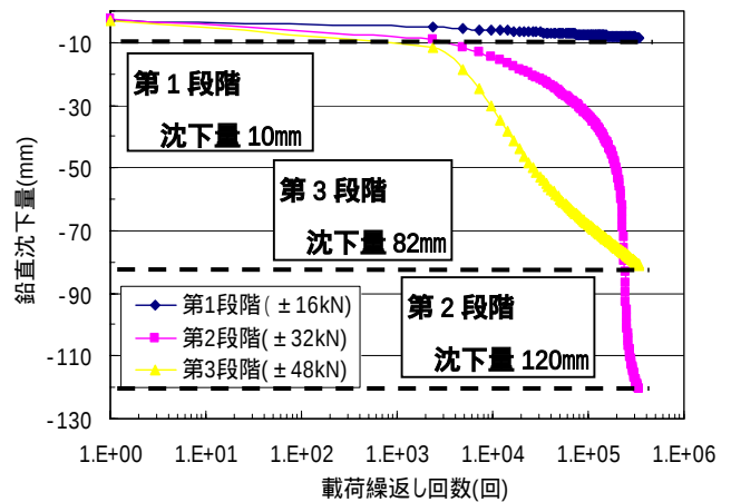
図5 繰返し回数と沈下量の関係 (直接基礎)
