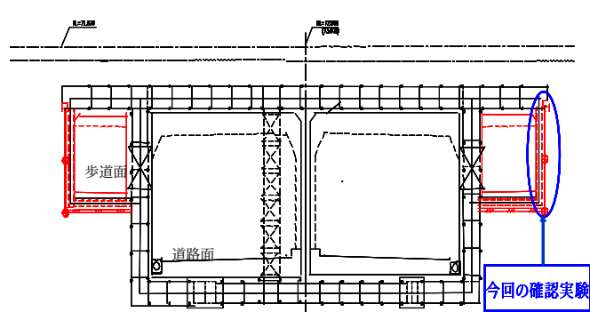
図-2 新しい施工法
