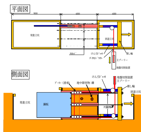
図-4 実地試験の平面図と断面図
