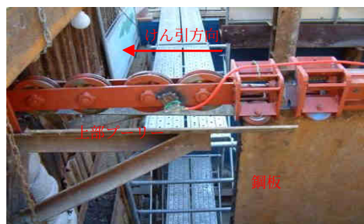
図-7 上部プーリー設置状況
