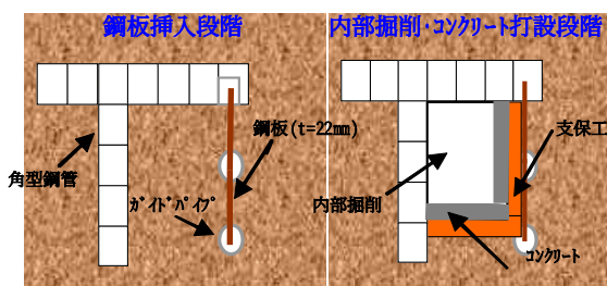
図-3 鋼板挿入の施工ステップ
