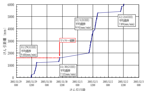
図-5 実験進捗図
