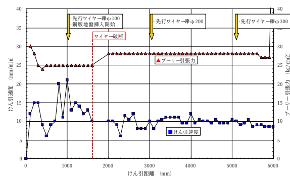
図-6 けん引速度とプーリー軸トルク
