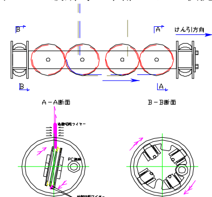
図-9 プーリーが傾いた状況
