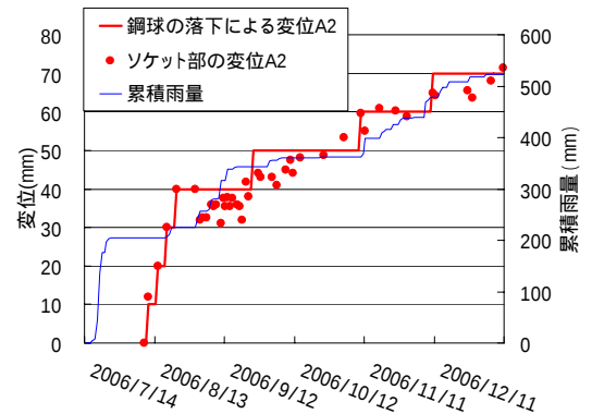
図-4 装置A2の計測結果
