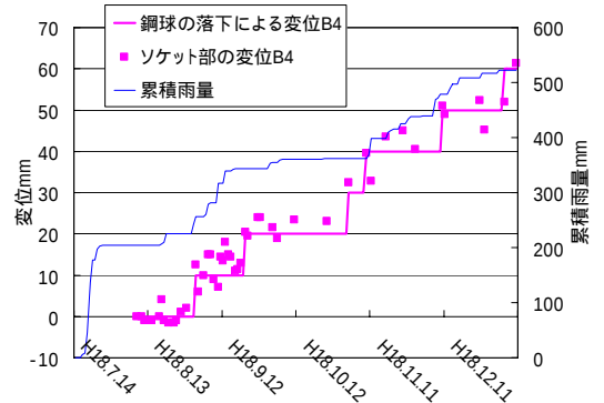
図-5 装置B4の計測結果
