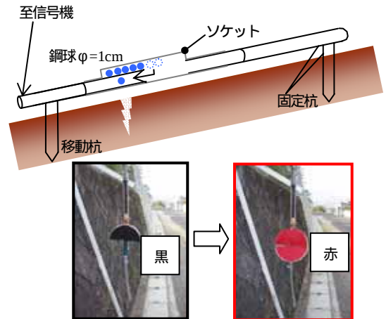
図-1 住民参加型斜面監視装置の概要
