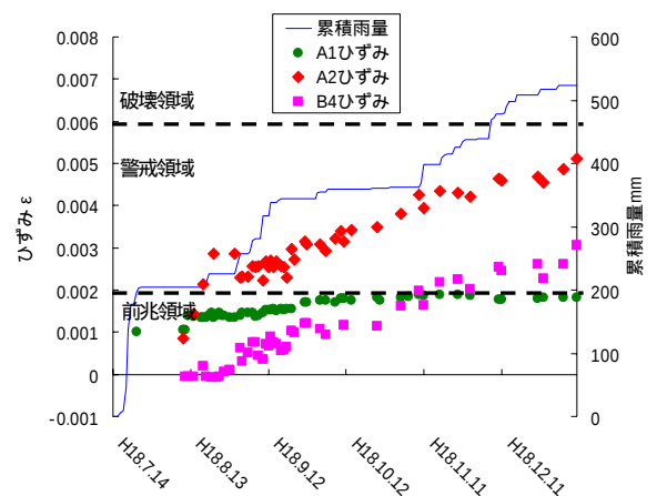
図-6 時間変位によるひずみ量
