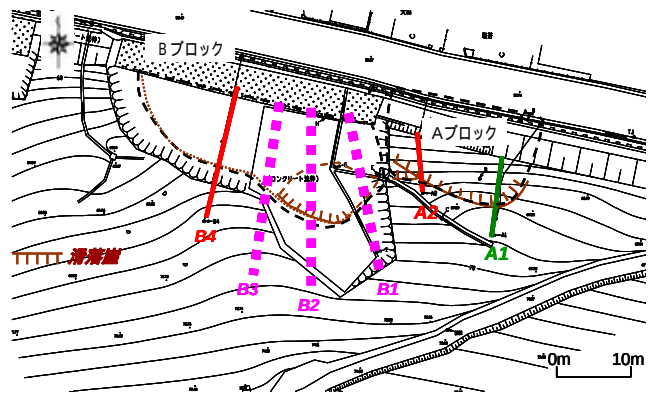
図-2 斜面装置の配置図
