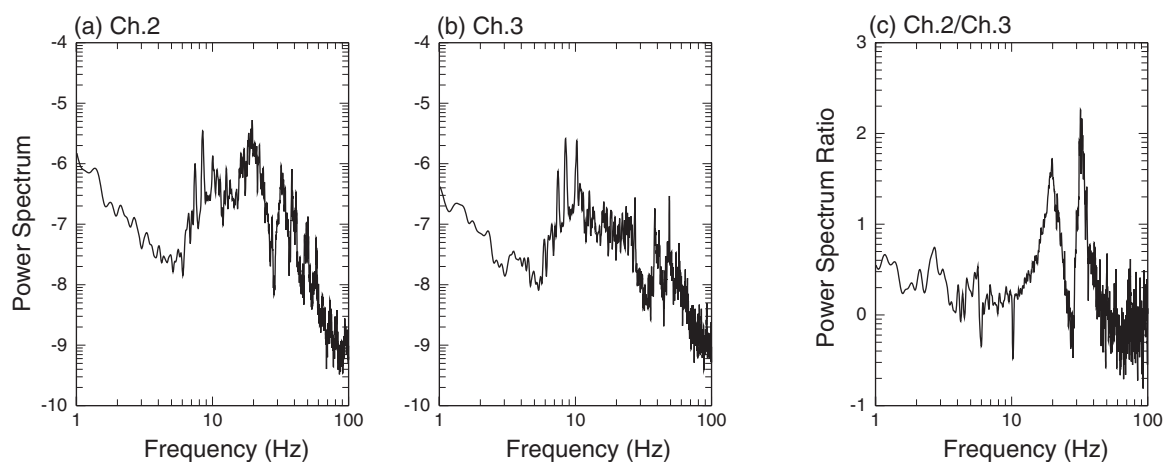
図-2 Site A におけるパワースペクトルとパワースペクトル比。(a) 不安定な岩塊上のスペクトル (Ch.2), (b) 基盤上のスペクトル (Ch.3), (c) 岩塊上／基盤上のスペクトル比
