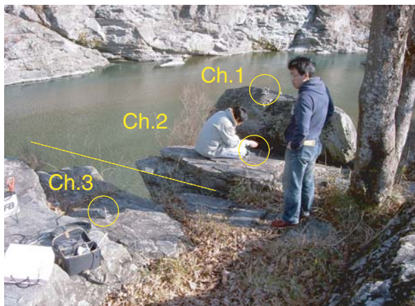
図-1 常時微動の観測状況。(a) Site A (不安定と考えられる岩塊), (b) Site B (安定と考えられる岩塊)
