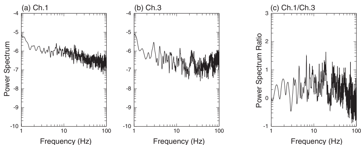
図-3 Site B におけるパワースペクトルとパワースペクトル比。(a) 安定な岩塊上のスペクトル (Ch.1), (b) 基盤上のスペクトル (Ch.3), (c) 岩塊上／基盤上のスペクトル比
