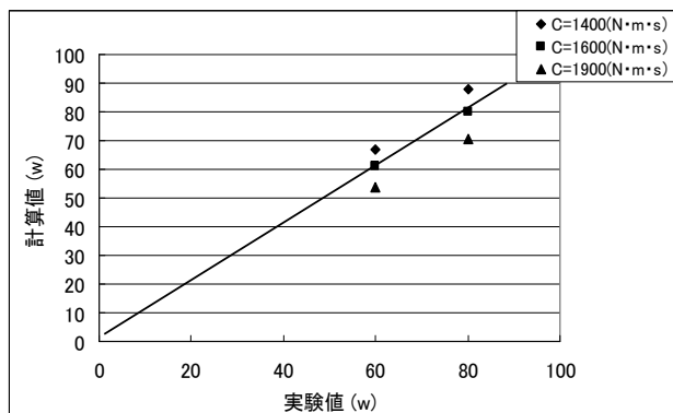
図-3 粘性減衰係数 C の決定
