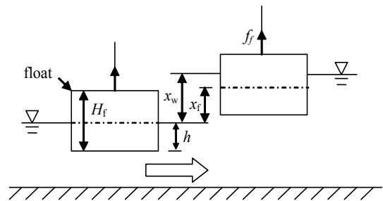
図-2 フロートの変位
