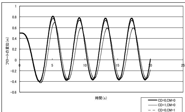
図-5 フロートの変位と C_D , C_M の関係
