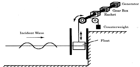
図-1 動力変換の全体のシステム
