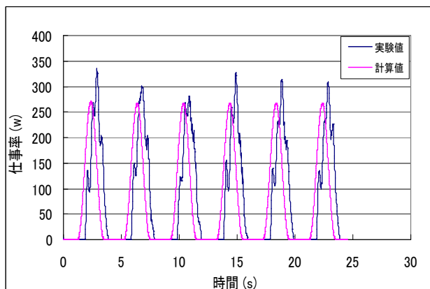
実験 1
