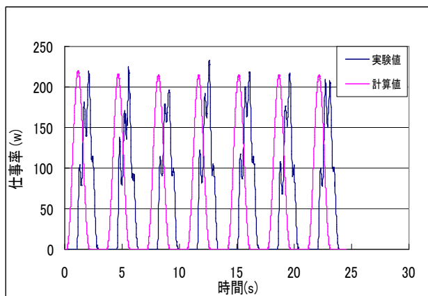
実験 2
