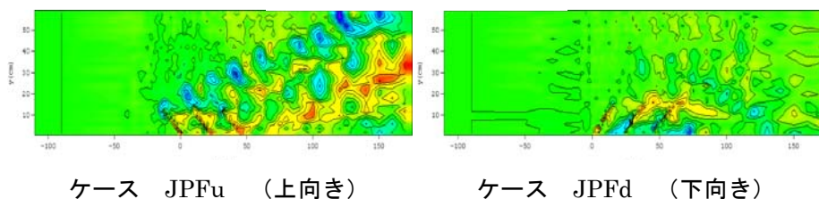
図-3 水制設置角度による影響を調べるための河床高コンター
