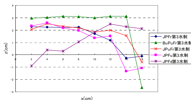
図-2 第3水制形状図
