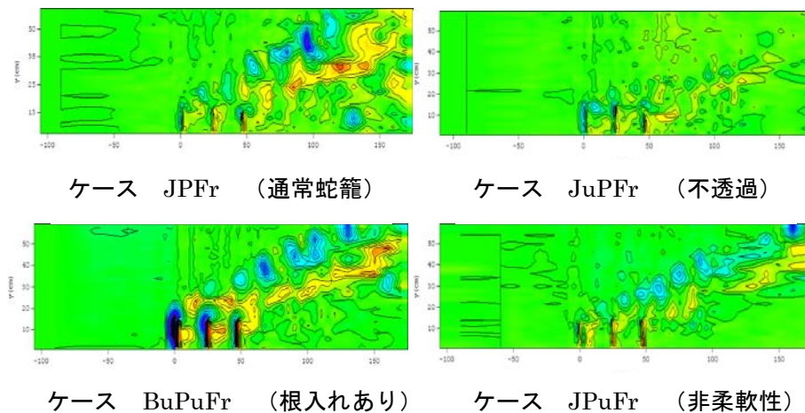
図-1 蛇籠の物理的特性を変えた影響を調べるための河床高コンター
