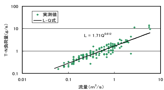
図5 L-Q 式(T-N)
