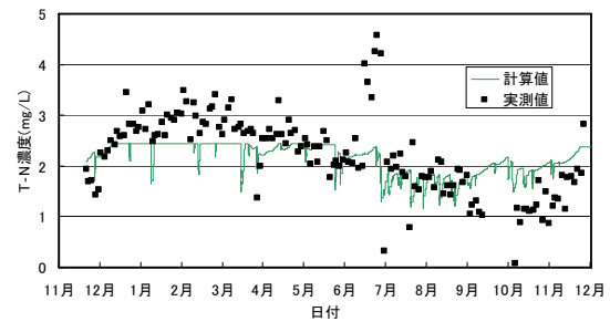
図7 T-N 濃度の推定
