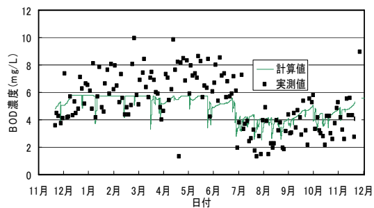
図6 BOD 濃度の推定
