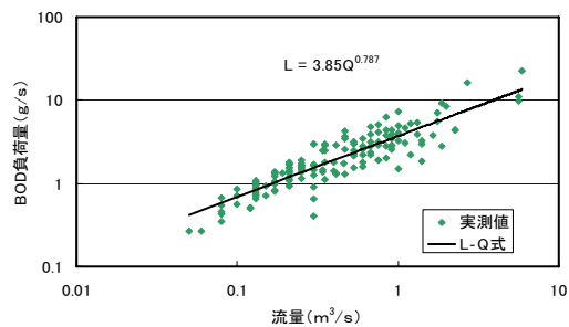
図4 L-Q 式(BOD)
