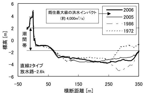
図4 干潟横断面の経年変化
