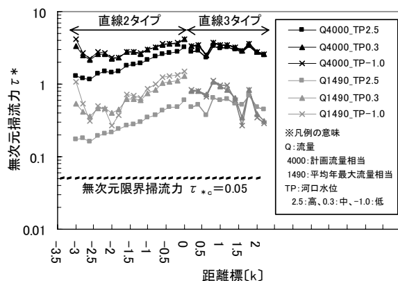
図5 洪水時に干潟に作用する無次元掃流力と無次元限界掃流力の関係
