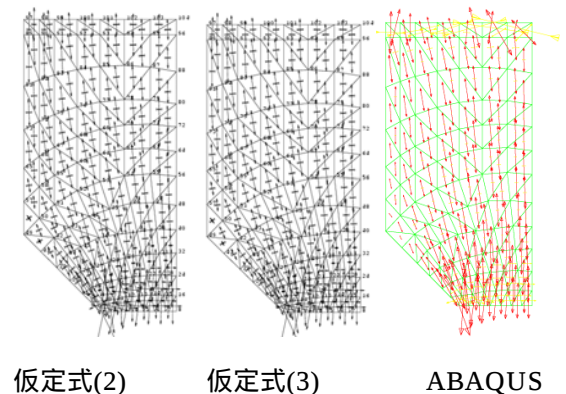
Fig.4 P=6.3\text{kN} 時の応力分布
