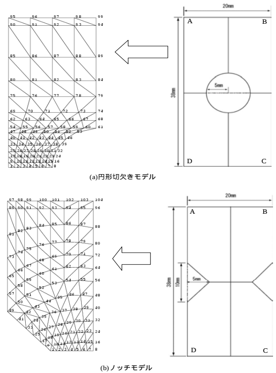
Fig.2 解析対象モデルとメッシュ
