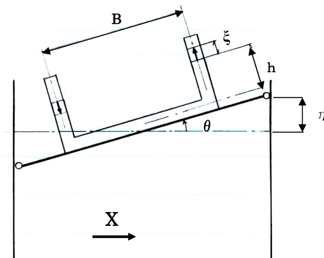
図-2 浮屋根スロッシングへの TLCD の適用
