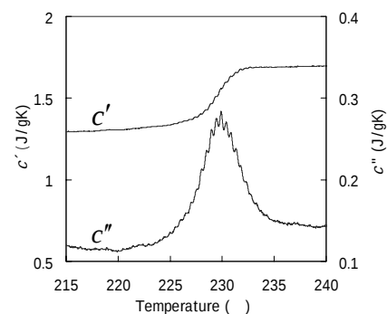
図-2 複素比熱測定
