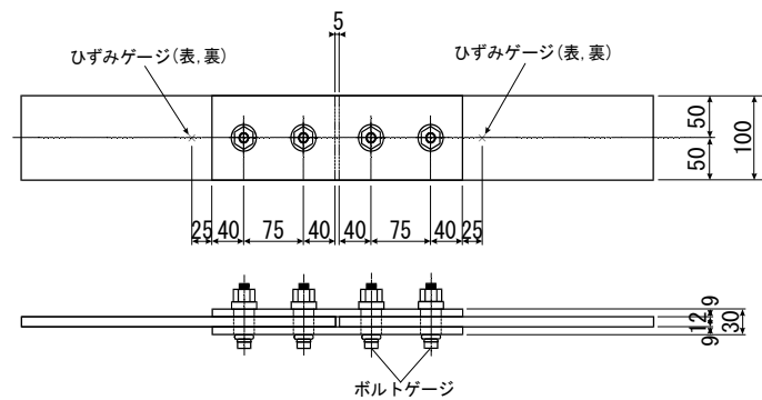
図-4. 試験体形状
