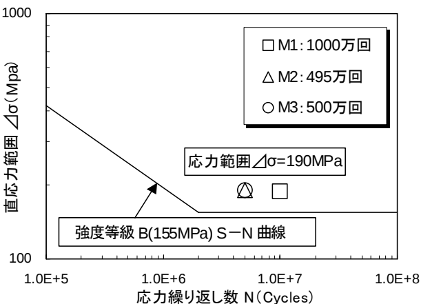
図-5. 疲労試験結果
