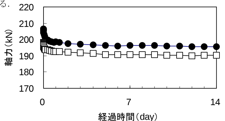
図-3. 軸力リラクセーション試験結果
