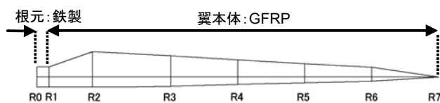
図3 翼の形状
