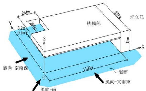
図 - 2 栈橋解析モデルと風向
