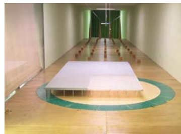
写真-1 栈橋部実験模型
