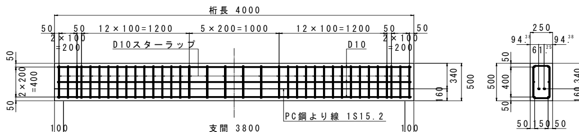
図 1 供試体形状寸法
