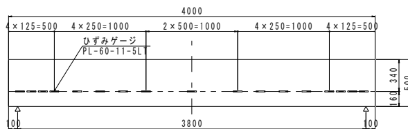
図 2 ひずみゲージ貼付位置
