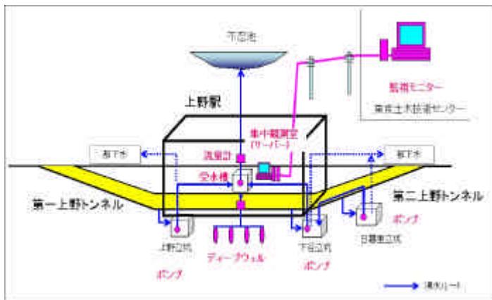
図-2 上野駅隣接トンネルからの湧水ルートと湧水処理システム
