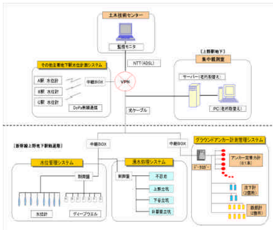
図-4 上野駅維持管理システム略図
