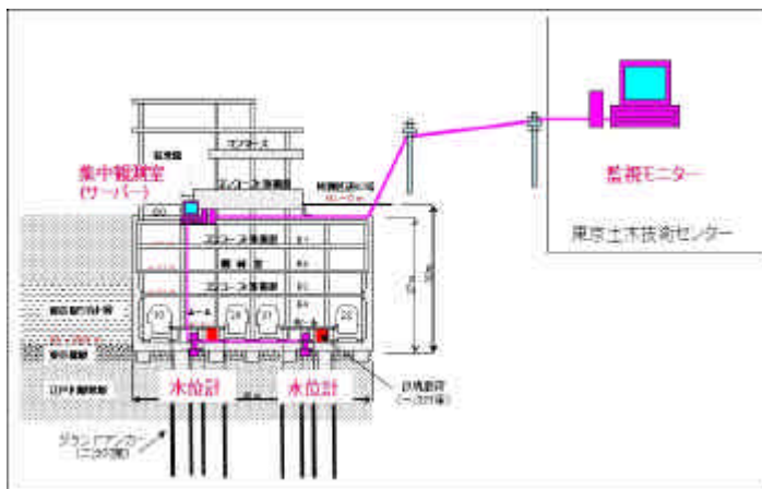
図-1 上野駅断面図及び水位管理システム
