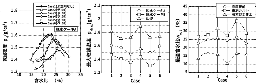
図-3 締固め曲線
