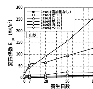
図-14 E_{50} と養生の関係
