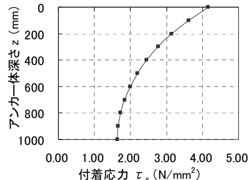
図-5 付着応力度分布 (case1-3)
