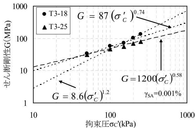
図-3 G \sim \sigma_c' の関係
