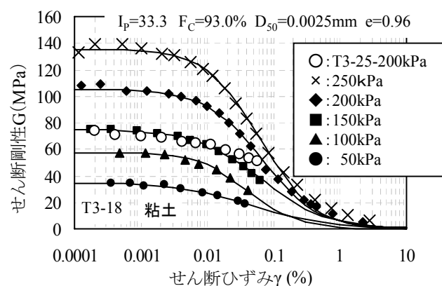
図-2 G ～ \gamma の関係
