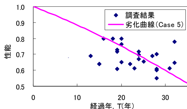
図-2 劣化曲線の妥当性の検証
