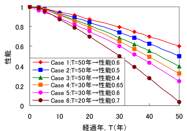
図-1 基本劣化曲線
