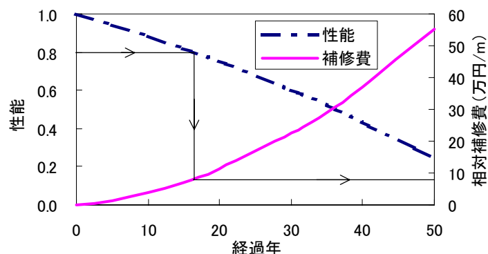
図-3 性能に対する相対補修費
