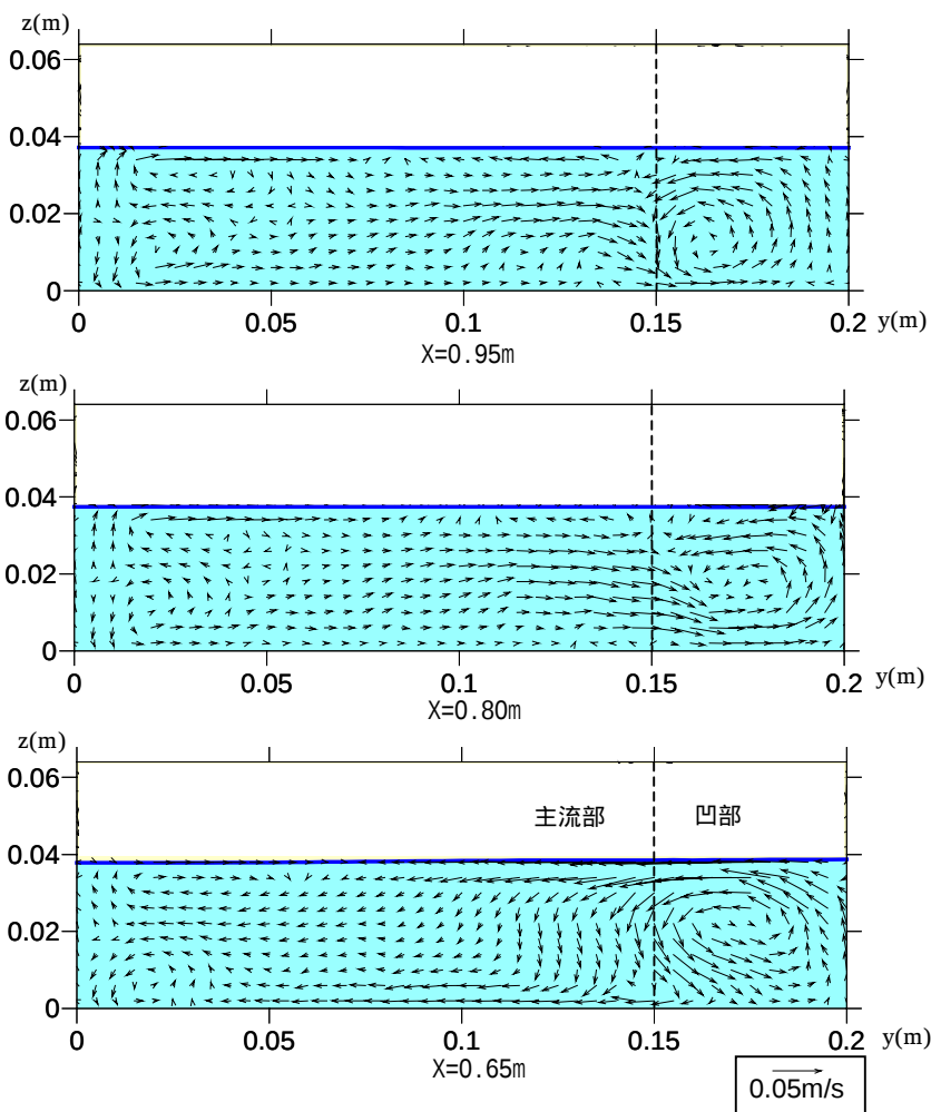
図-3 凹部内横断面の流速分布 ( Fr=0.8 )
