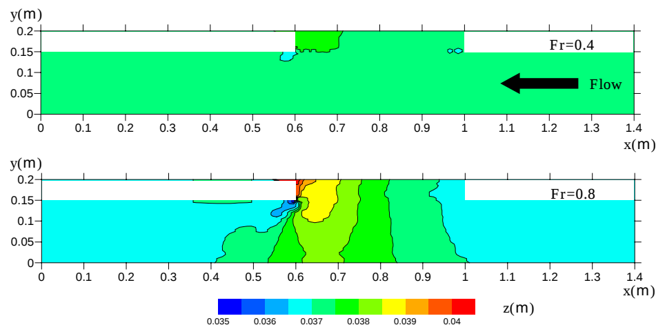
図-1 解析結果の時間平均水深分布
