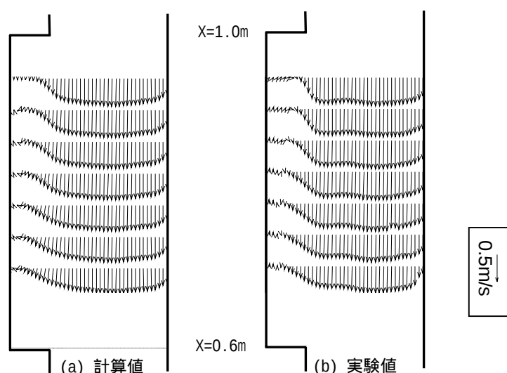
図-2 実験における流速分布との比較 ( Fr=0.8 Z=0.01\text{m} )
