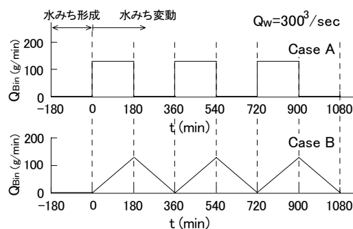
図-1 給砂条件
