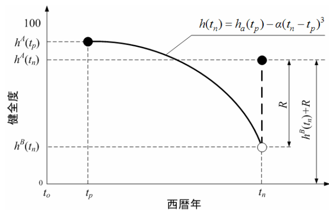
図 1 劣化曲線と対策効果
