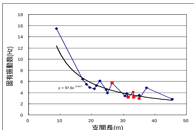
図—2 支間長—固有振動数
