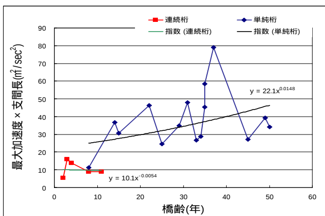
図—5 橋齢—最大加速度 \times 支間長
