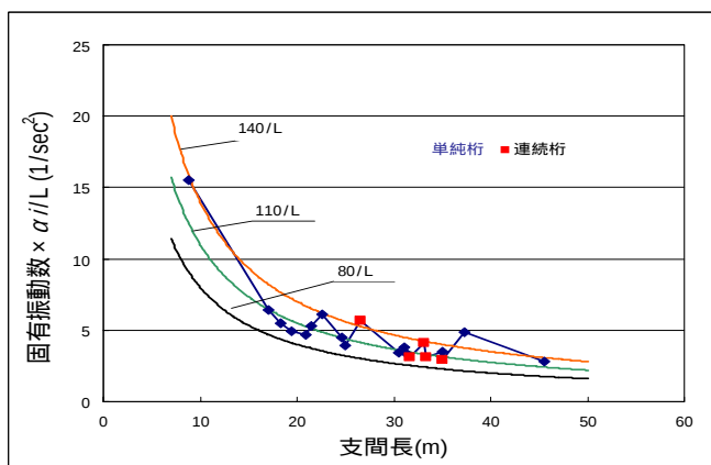
図—3 支間長—固有振動数 \times \alpha i / L
