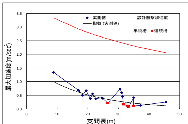
図—1 支間長—最大加速度
