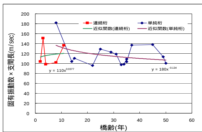
図—4 橋齢—固有振動数 \times 支間長
