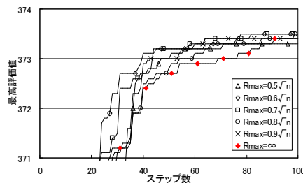
図-6 群最良値の収束状況に及ぼす探索範囲制約の効果
