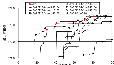
図-7 局所ランダム探索が最良値探索に及ぼす影響
