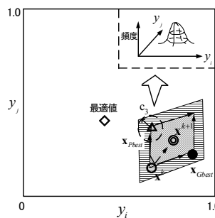
図-4 局所ランダム探索機能説明図
