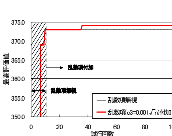
図-8 局所ランダム項を途中から付加した場合
