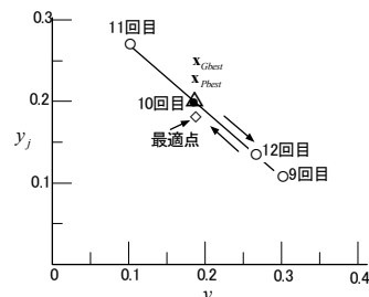
図-9 局所ランダム項を途中から付加したもの
