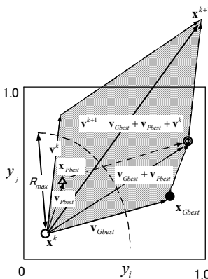
図-3 探索域制約の説明
