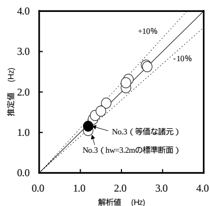
図 - 1 鉛直たわみ基本振動数の対比
