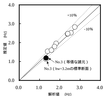
図 - 2 ねじれ基本振動数の対比
