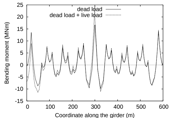
図-5 斜張橋の桁の曲げモーメント
