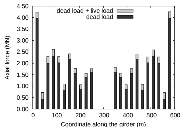
図-6 斜張橋のケーブルの軸力
