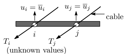
図-1 ケーブル張力（プレストレス力）
