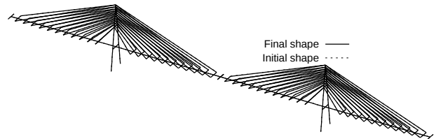
図-4 斜張橋の形状決定後の形状
