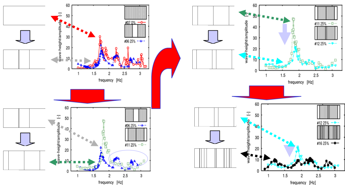
図 3 遮閉板の改良
