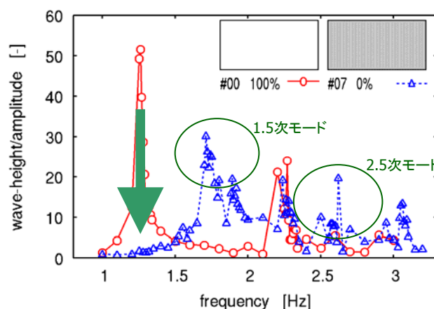
図2 遮閉板によるスロッシング防止効果
