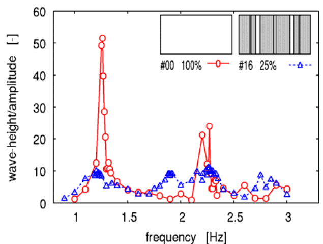
図 4 改良後の応答関数
