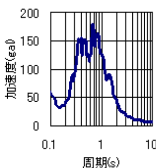
(a) 神戸波
