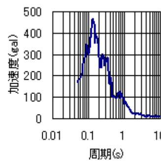
(b) 芸予波
