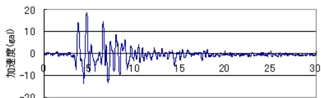
(a) 神戸波
