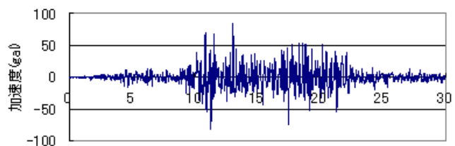
(b) 芸予波
