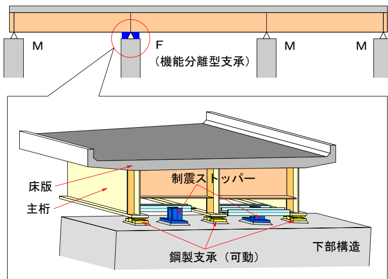
図-1 制震ストッパーの適用例
