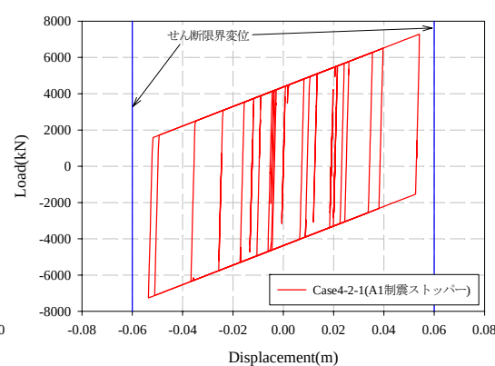
(b) 荷重-変位関係
