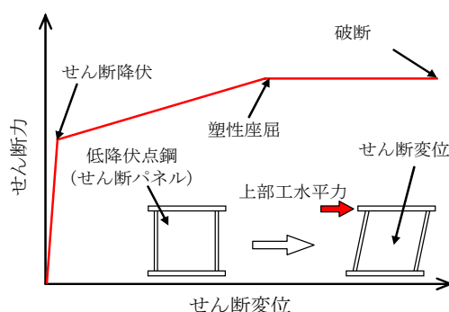
図-2 制震ストッパーの非線形特性
