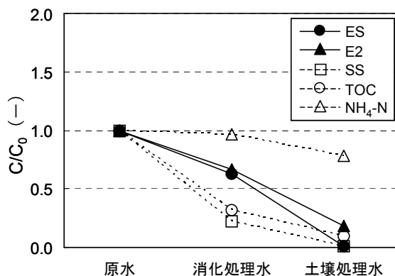
図-2 原水貯留槽流入部における原水に対する消化処理水および土壤処理水の比
