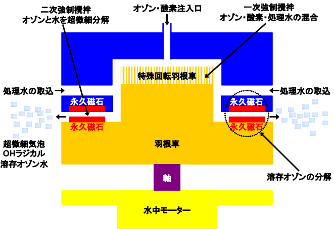
図-1 オゾン・磁場・超微細気泡併用型水質浄化装置
