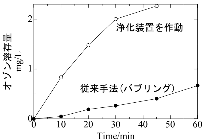
図-2 オゾン水溶解性試験結果
