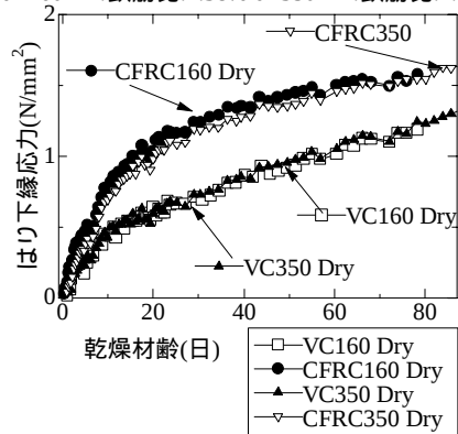
図5 拘束応力
