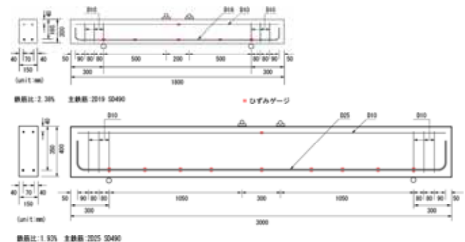
図 1 供試体概要
