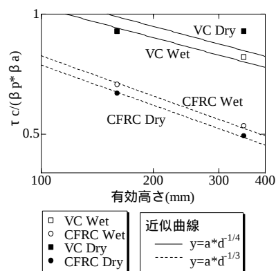
図7 寸法効果
