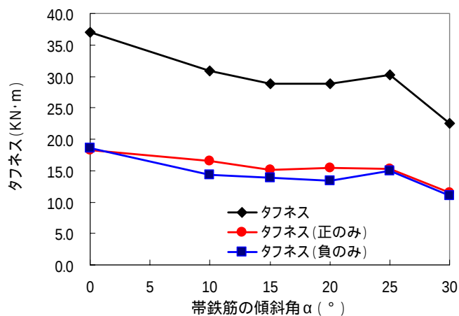
図-4 タフネスと傾斜角の関係
