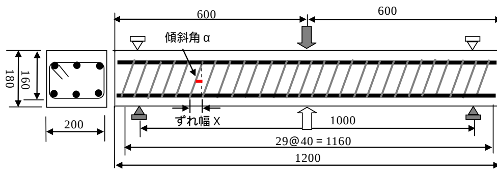
図-1 供試体寸法の例
