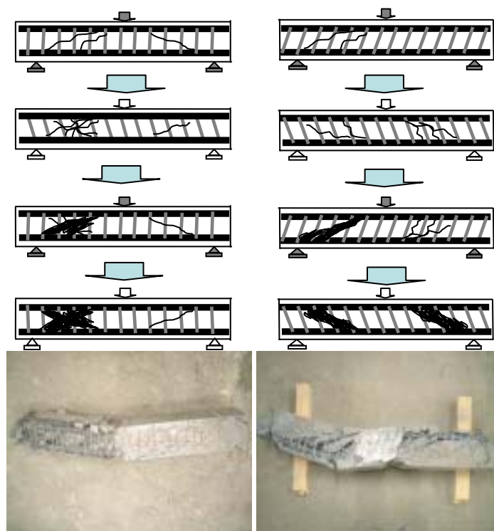
(a) \alpha が 0^\circ および 10^\circ の場合 (b) \alpha が 15^\circ 、 25^\circ および 30^\circ の場合
