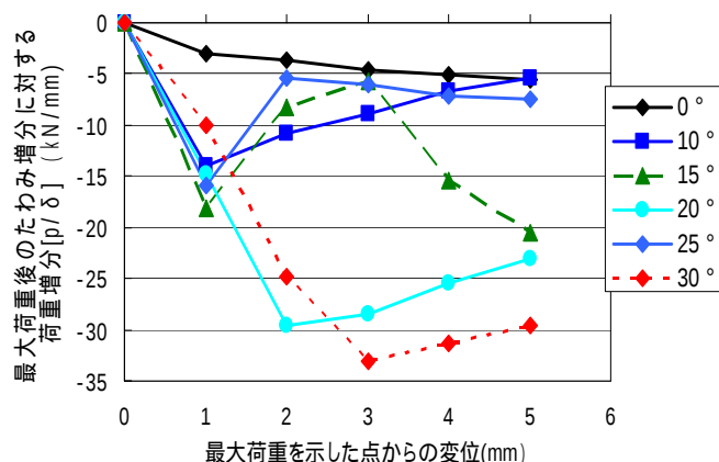
図-5 2回目の正方向時の最大荷重からの変位と傾きの関係
