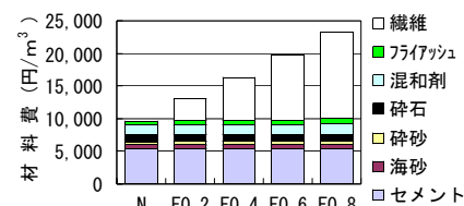
図-6 各配合とコンクリート材料費
