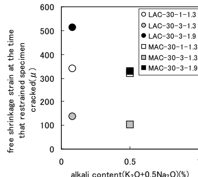
図-2 モルタルにおけるひび割れ発生時の自由収縮ひずみ量とアルカリ含有量の関係
