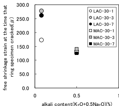
図-1 セメントペーストにおけるひび割れ発生時の自由収縮ひずみ量とアルカリ含有量の関係
