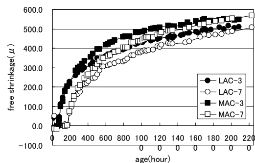
図-5 自由収縮ひずみ量と材齢の関係
