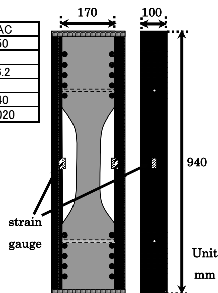
図-3 一軸拘束ひび割れ試験型枠
