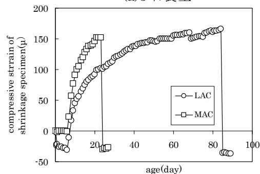
(b)7 日養生
