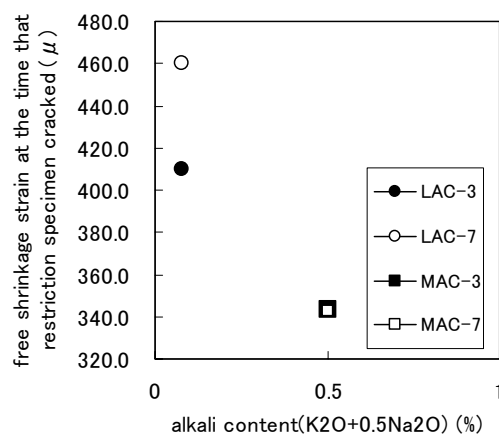
図-6 ひび割れ発生時の自由収縮ひずみ量とアルカリ含有量の関係
