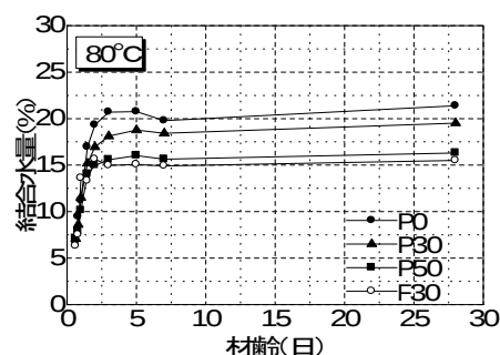
図-4 結合水量の経時変化 (80℃養生)
