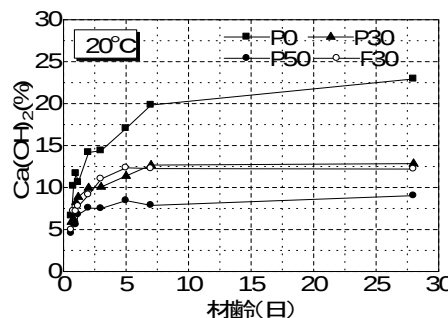
図-5 \text{Ca}(\text{OH})_2 量の経時変化 (20℃養生)
