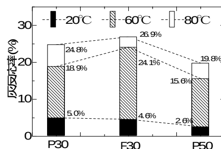
図-8 材齢 28 日における灰反応率
