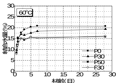
図-3 結合水量の経時変化 (60℃養生)
